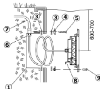
Vgradnja v plastični ali kovinski bazen
