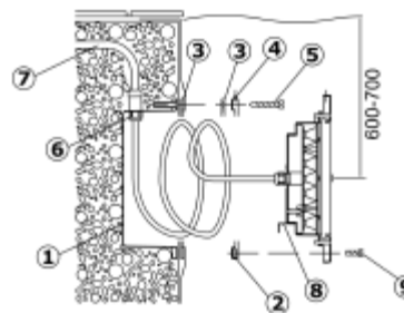
Vgradnja v beton - folija
