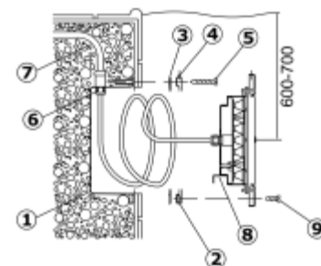
Vgradnja v beton - keramiko
