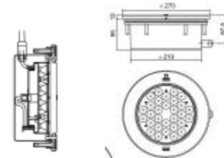
Vgradnja v beton - keramiko
